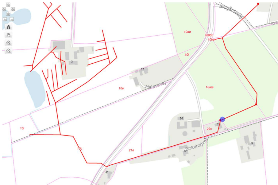
Figur 1: de røde linjer markerer placering af dræn, den blå cirkel markerer stedet for krydsning.
